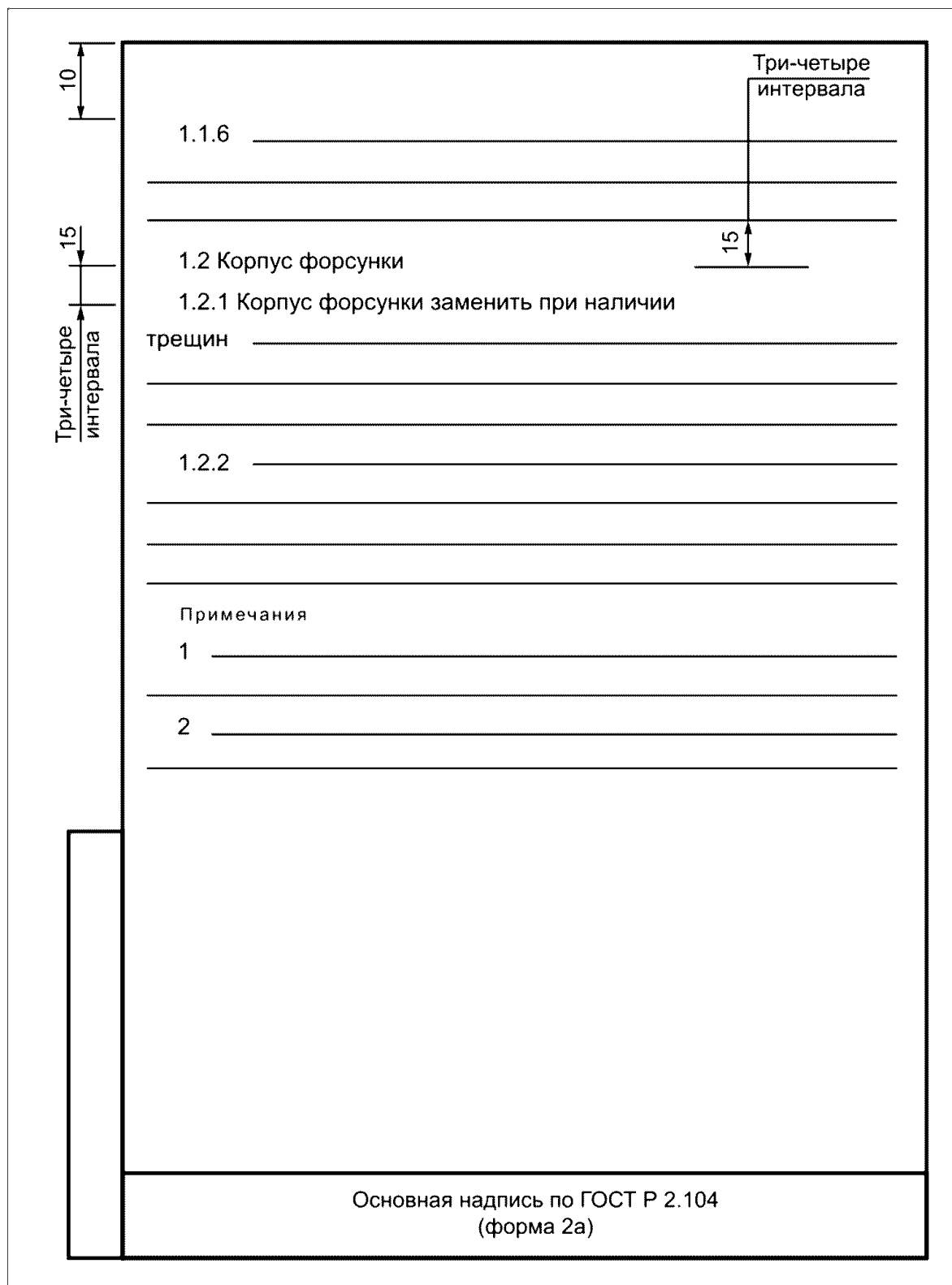
Рисунок А.2 - Пример выполнения последующих листов ТД
