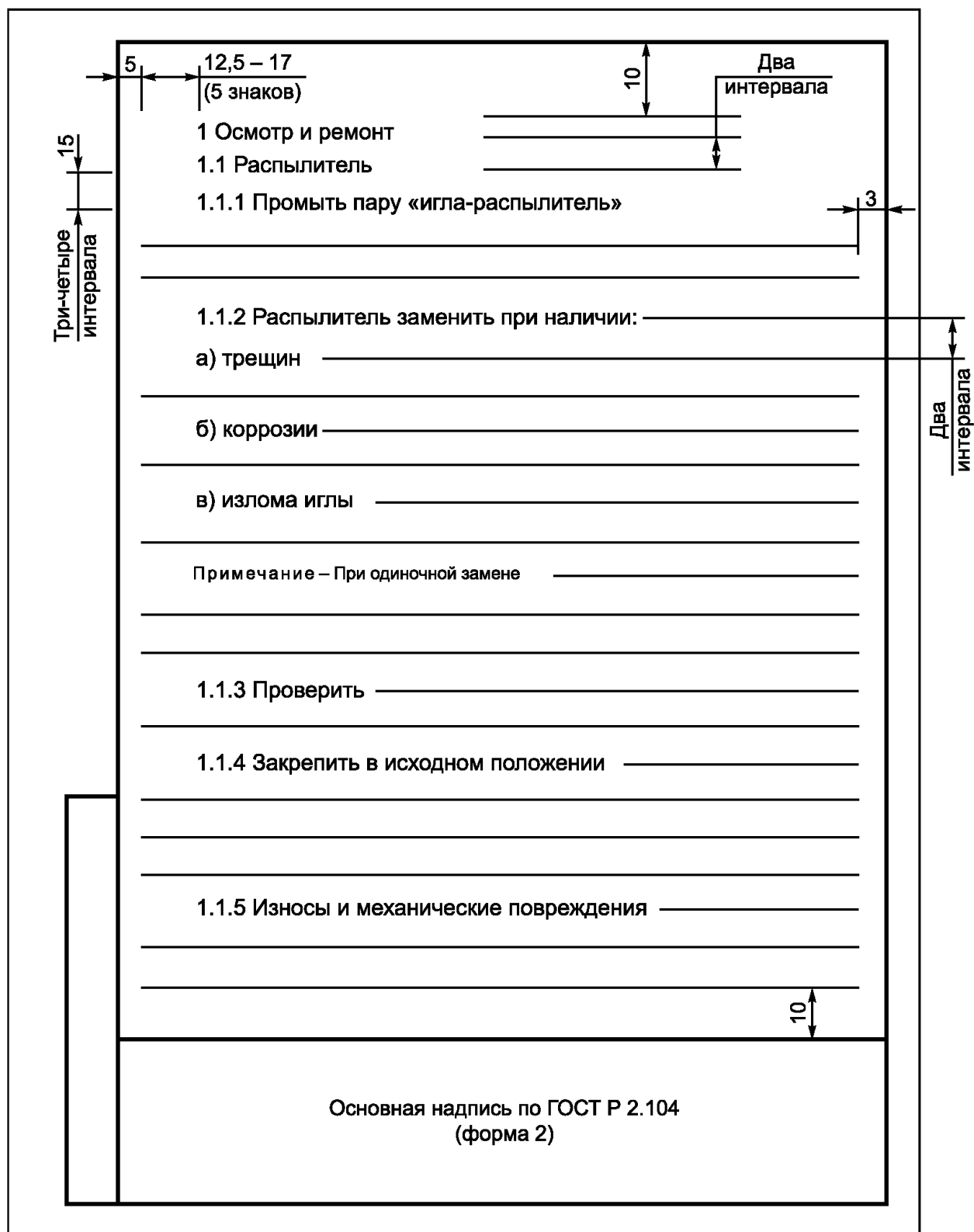
Рисунок А.1 - Пример выполнения первого нумеруемого листа ТД с основной надписью
